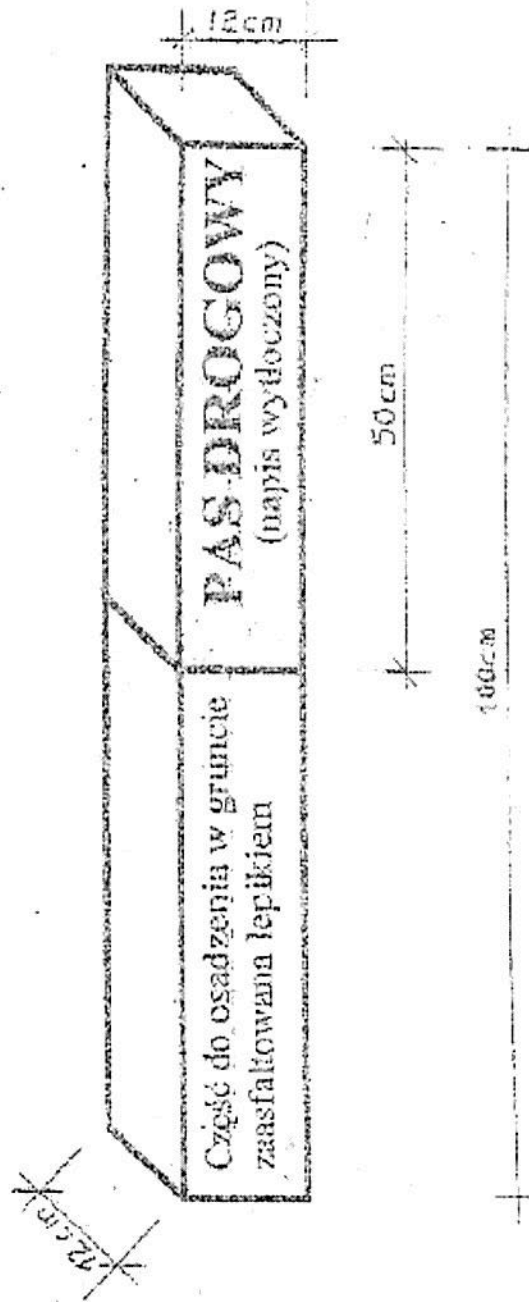
(Rys. 1) Świadek punktu granicznego w części nadziemnej z każdej strony pomalowany na żółto farbą choroekauczkową z czarnym napisem, wykonany z betonu B-25 zbrojonego 4 prętami \varnothing 10
