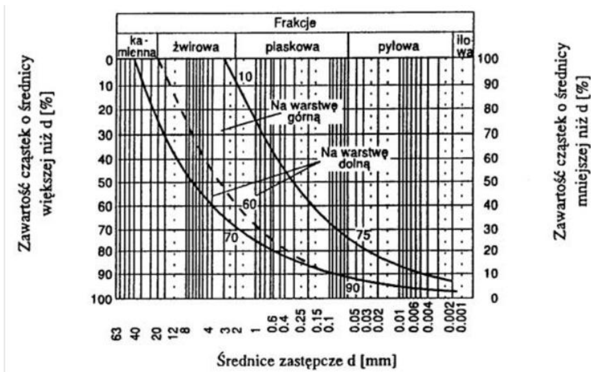
Rys. 2. Obszar uziarnienia optymalnej mieszanki gliniasto-żwirowej
