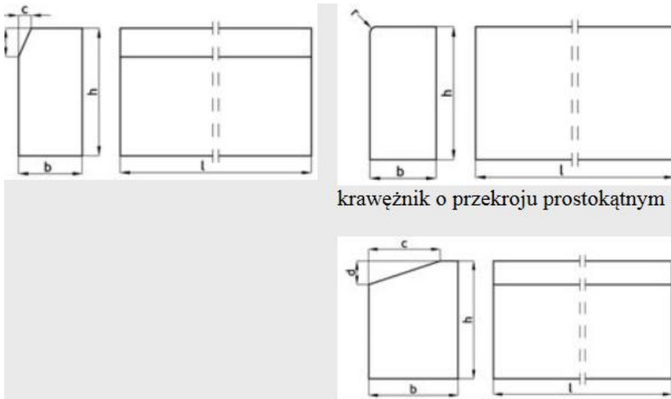
Przykładowe wymiary krawężników
