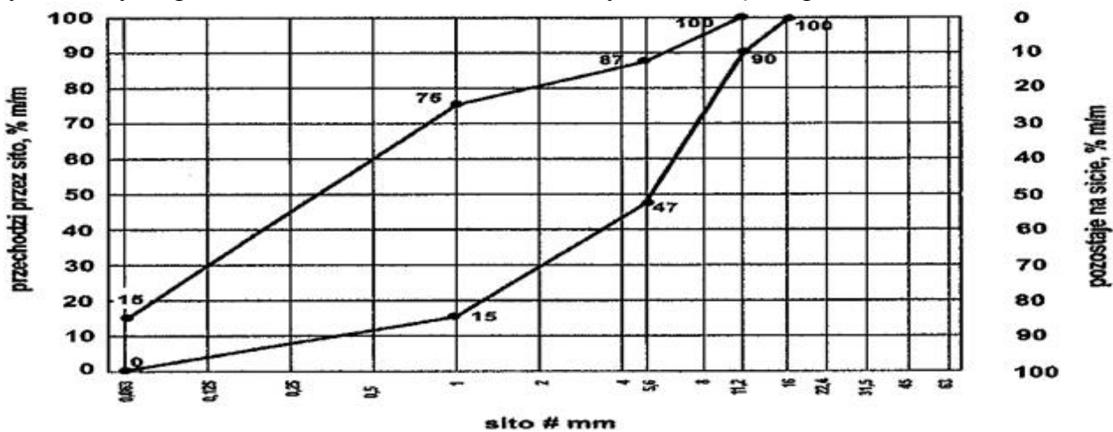
Rys. 2. Krzywe graniczne uziarnienia mieszanki kruszywa niezwiązanego 0/11,2 mm do nawierzchni
