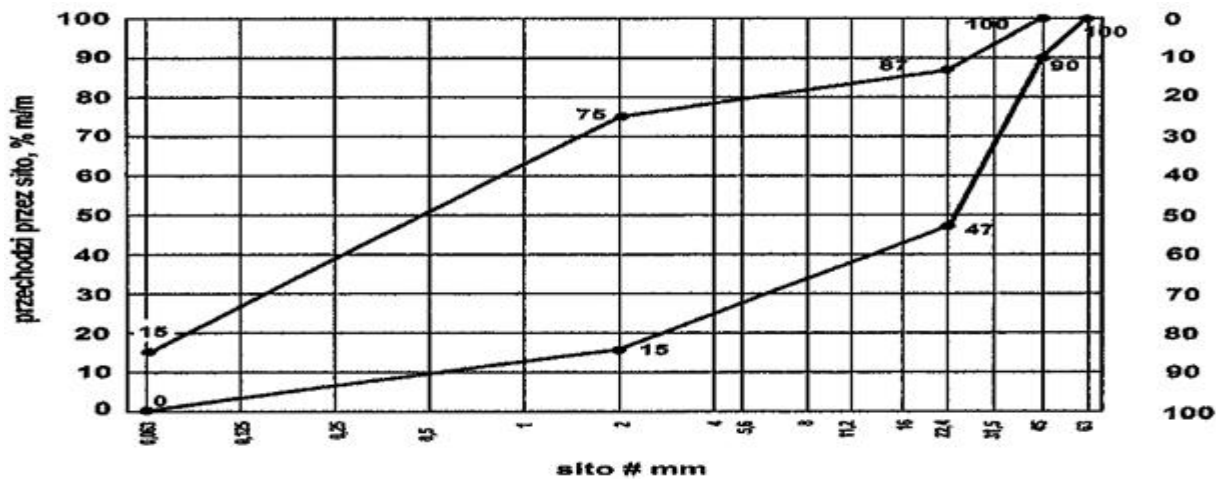
Rys. 6. Krzywe graniczne uziarnienia mieszanki kruszywa niezwiązanego 0/45 mm do nawierzchni
