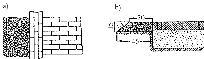
Rys. 4. Obramowanie jezdni z trzech rzędów klinkieru z umocowaniem warstwą tłucznia a) widok z góry b) przekrój poprzeczny
