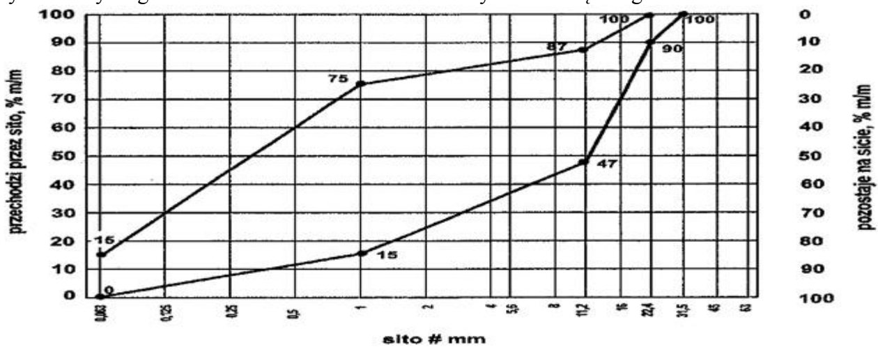
Rys. 4. Krzywe graniczne uziarnienia mieszanki kruszywa niezwiązanego 0/22,4 mm do nawierzchni
