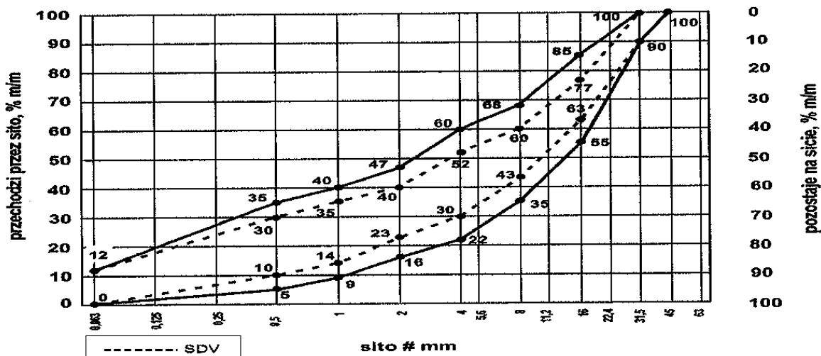
Rys. 1. Krzywe graniczne uziarnienia mieszanki kruszywa niezwiązanej 0/31,5 mm do warstw podbudowy pomocniczej
