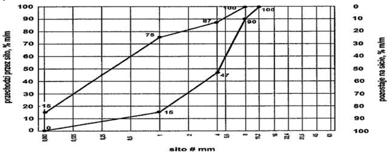
Rys. 1. Krzywe graniczne uziarnienia mieszanki kruszywa niezwiązanego 0/8 mm do nawierzchni
