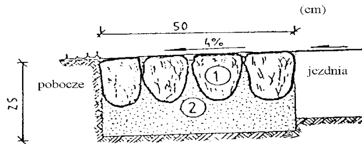
Rys. 1. Obramowanie jezdni z brukowca
