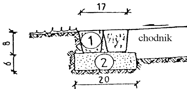
Rys. 2. Obramowanie chodników z kostki
