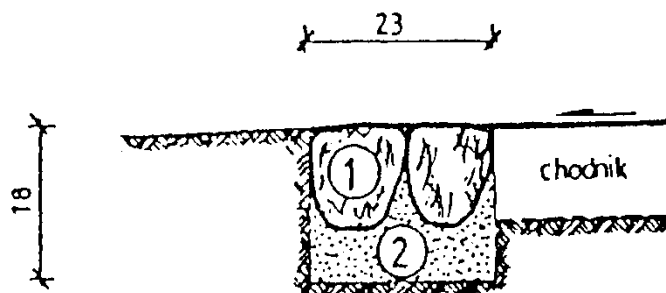
Rys. 3. Obramowanie chodnika z brukowca od 10 do 12 cm
