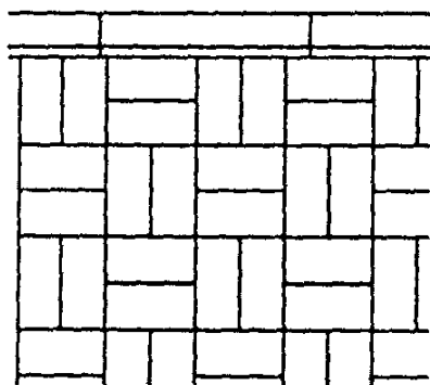
Rysunek 1 – deseń układania kostki (koszykowy).
