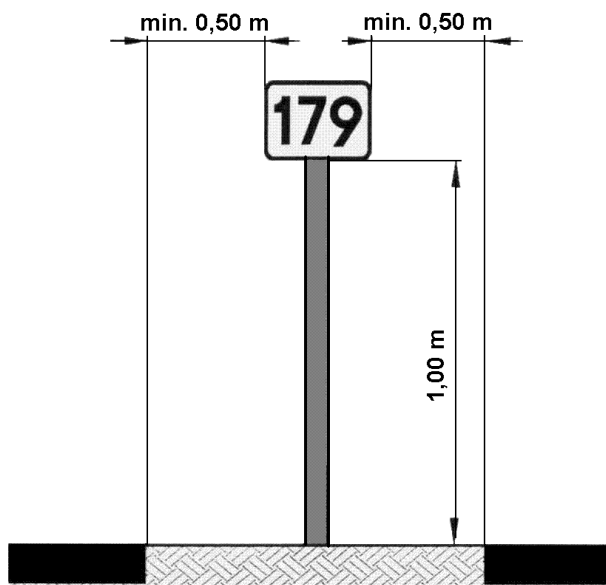
Rys. 3. Słupek krawędziowy U-2
