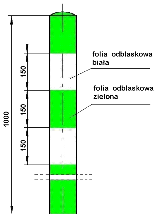
Rys. 3. Słupek krawędziowy U-2
