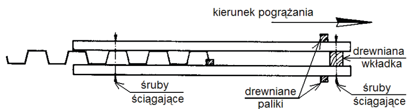
Stalowa rama prowadząca dla grodziec typu U
