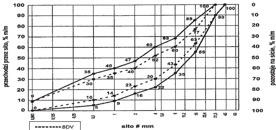
Rys. 2. Mieszanka niezwiązana 0/31,5 do warstwy podbudowy zasadniczej
