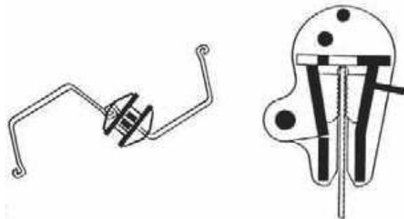
Rysunek 4. Przyrząd utrudniający wciąganie w grunt już pogrążonych w trakcie pogrążania następnej grodzicy.
