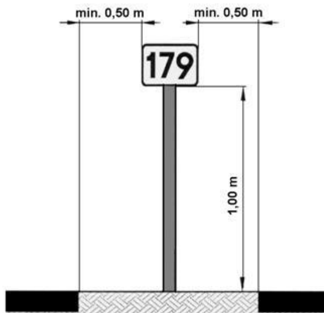
Rys. 4. Znak kilometrowy U-7 na samodzielny słupku
