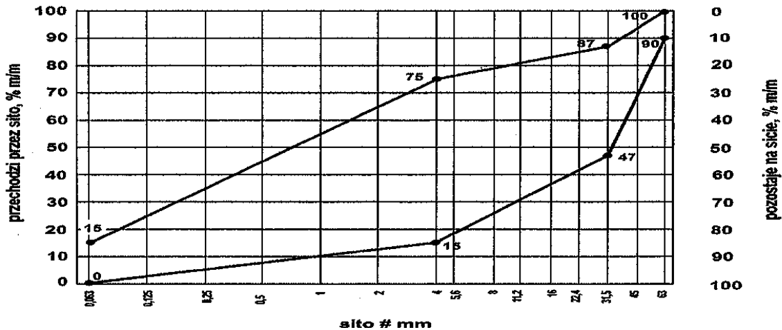
Rysunek 1. Uziarnienie mieszanki 0/63 do warstwy ulepszonego podłoża
