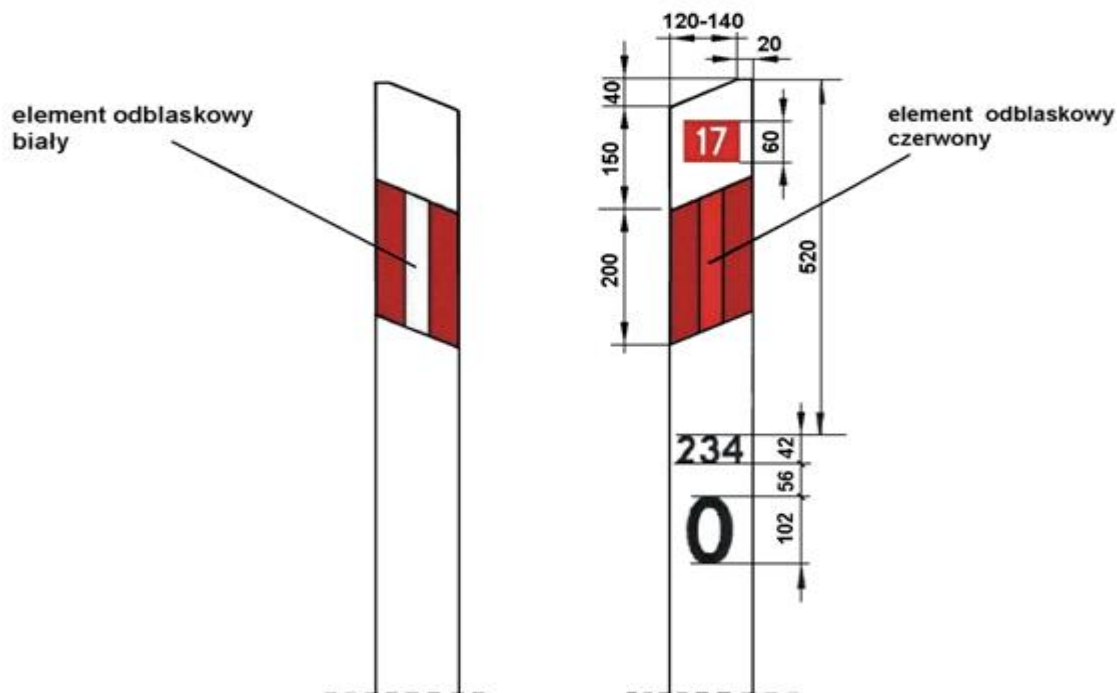
Rys.1. Słupek prowadzący U-1a z naniesionym numerem drogi, znakiem kilometrowym i hektometrowym, przeznaczony do umieszczenia na poboczu drogi, w hektometrze zerowym
