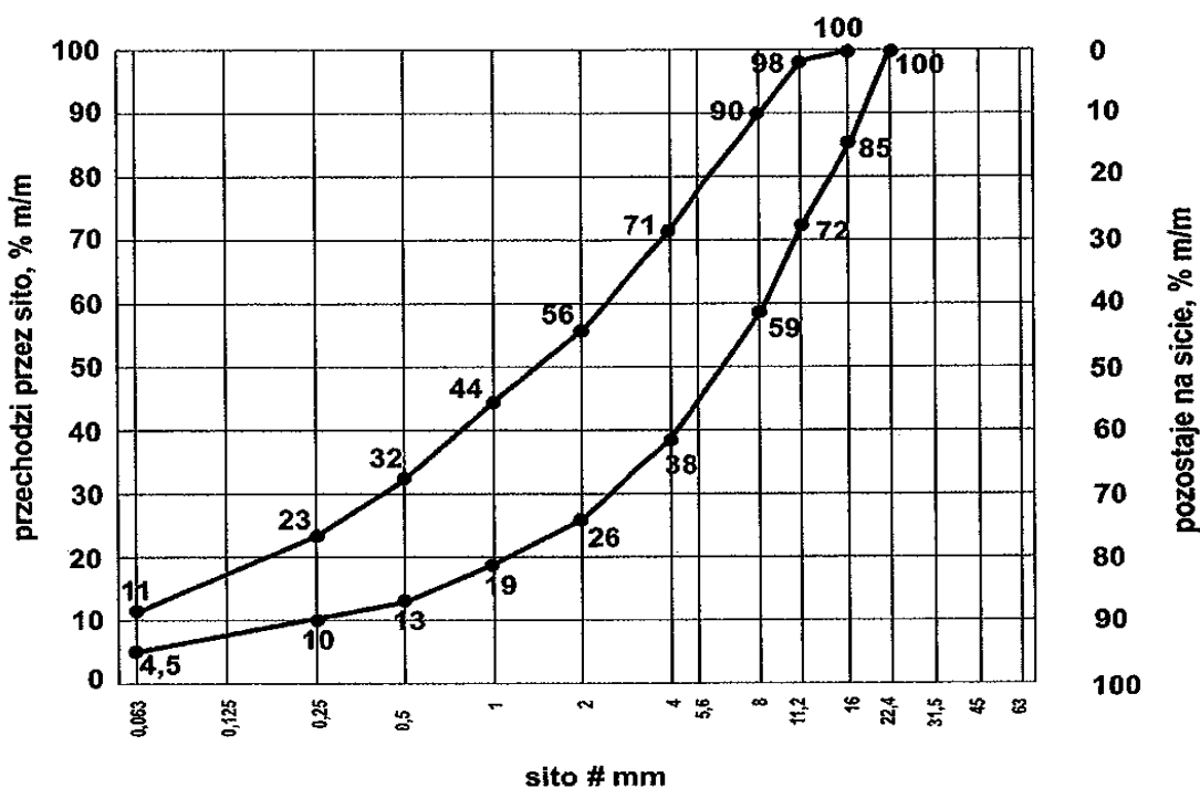
Rys. 3. Krzywe graniczne uziarnienia mieszanki mineralnej 0/16 mm
