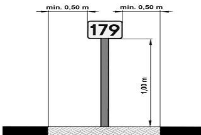
Rys. 3. Słupek krawędziowy U-2
