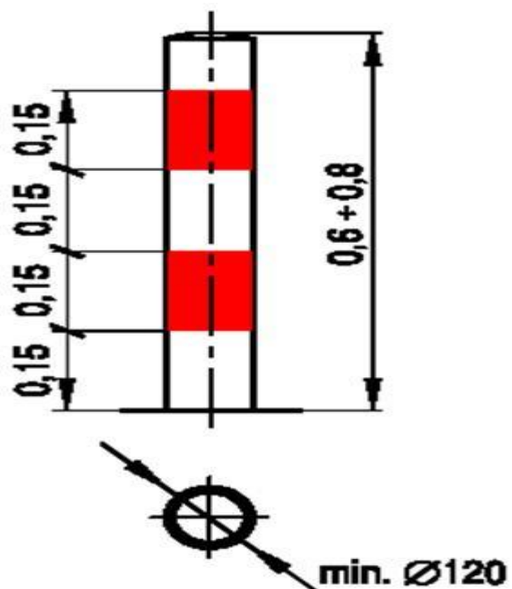
Rys. 5. Słupek blokujący U-12c
