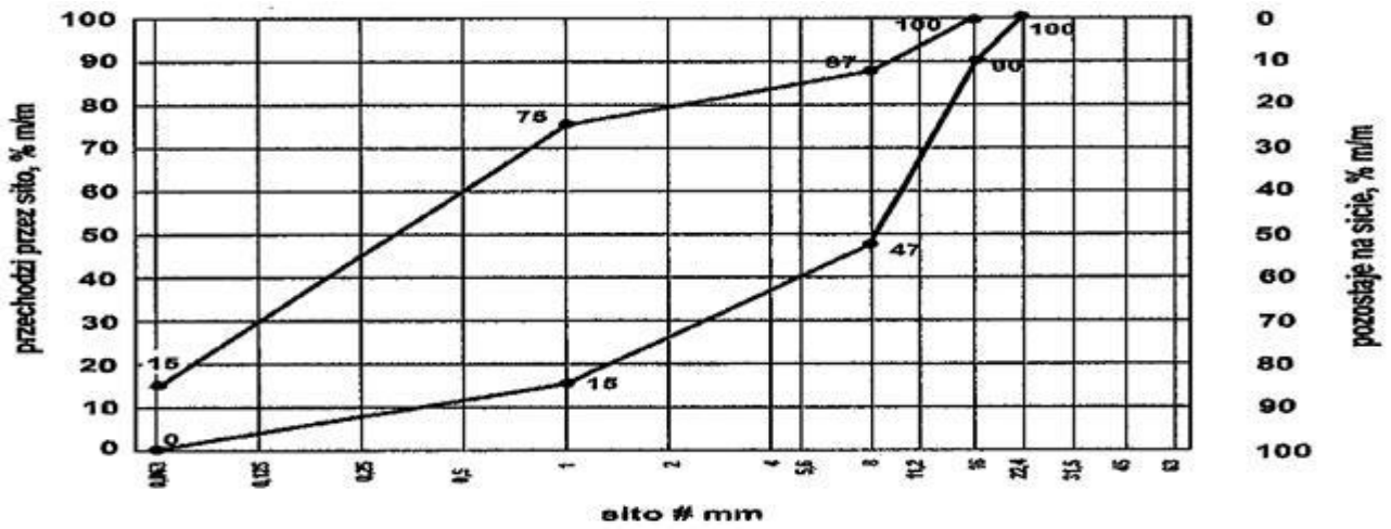
Rys. 3. Krzywe graniczne uziarnienia mieszanki kruszywa niezwiązanego 0/16 mm do nawierzchni
