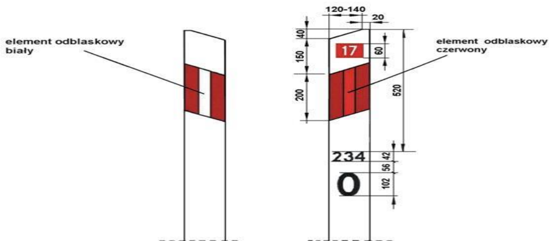
Rys.1. Słupki prowadzący U-1a z naniesionym numerem drogi, znakiem kilometrowym i hektometrowym, przeznaczony do umieszczenia na poboczu drogi, w hektometrze zerowym
