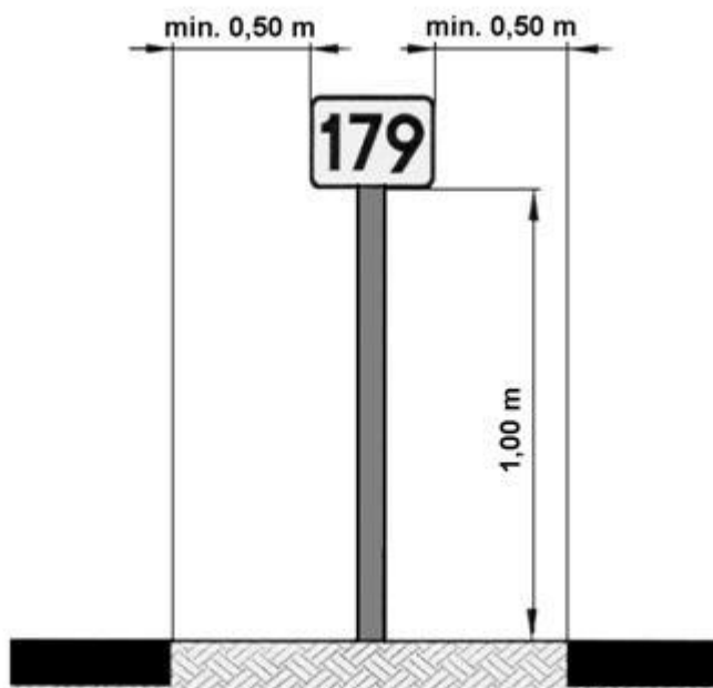
Rys. 3. Słupek krawędziowy U-2
