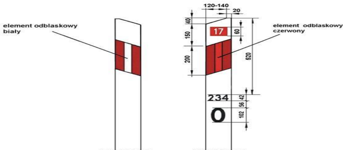
Rys.1. Słupek prowadzący U-1a z naniesionym numerem drogi, znakiem kilometrowym i hektometrowym, przeznaczony do umieszczenia na poboczu drogi, w hektometrze zerowym
