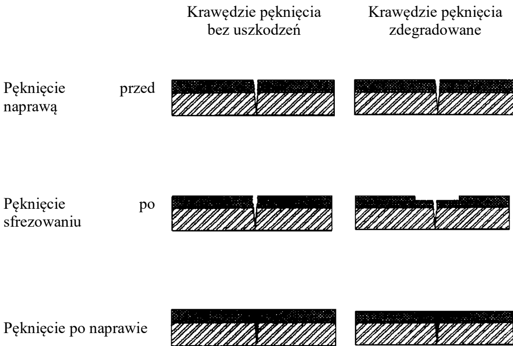
Rys. 2. Wypełnienie pęknięcia poszerzonego przez frezowanie
