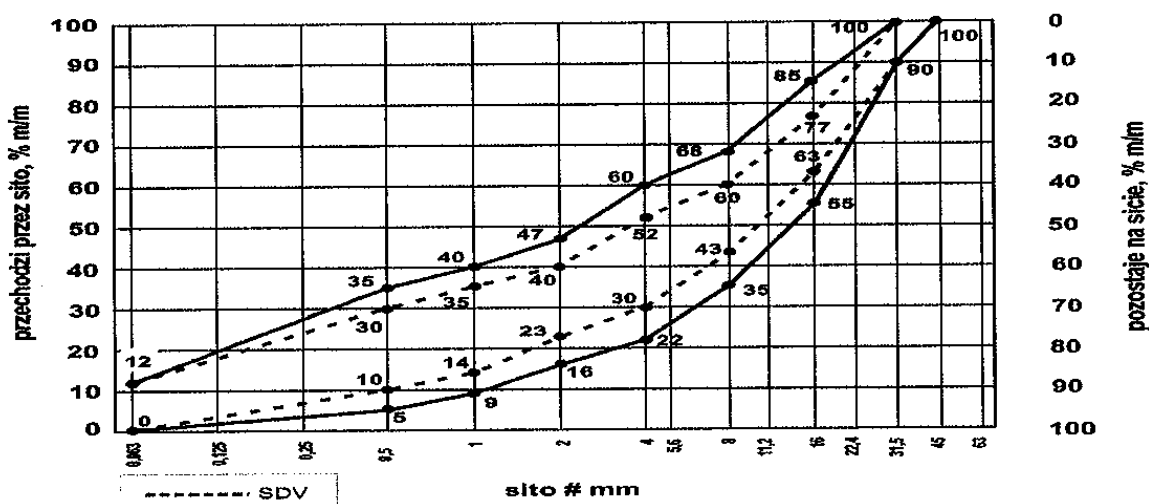
Rysunek 1. Uziarnienie mieszanki 0/31,5 do podbudowy pomocniczej oraz zasadniczej
