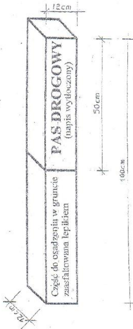
(Rys. 1) Świadek punktu granicznego w części nadziemnej z każdej strony pomalowany na żółto farbą chłoroekauczkową z czarnym napisem, wykonany z betonu B-25 zbrojonego 4 prętami \varnothing 10
