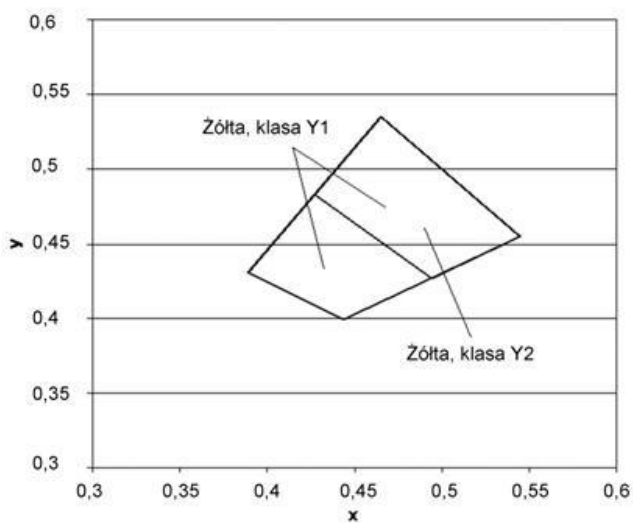
Tablica 11. Punkty narożne obszarów chromatyczności oznakowań dróg
