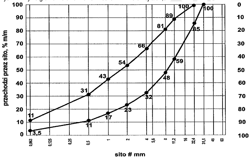
Rys. 2. Krzywe graniczne uziarnienia mieszanki mineralnej 0/22,4 mm
