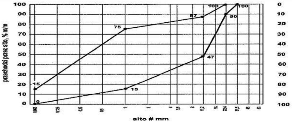
Rys. 4. Krzywe graniczne uziarnienia mieszanki kruszywa niezwiązanego 0/22,4 mm do nawierzchni
