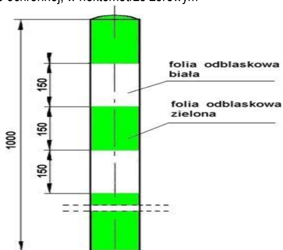
Rys. 2. Słupek prowadzący U-1b z naniesionym znakiem kilometrowym i hektometrowym, przeznaczony do umieszczenia na barierze ochronnej, w hektometrze zerowym
