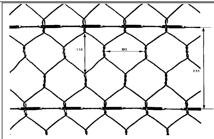
Rys. 1. Siatka z drutu stalowego
