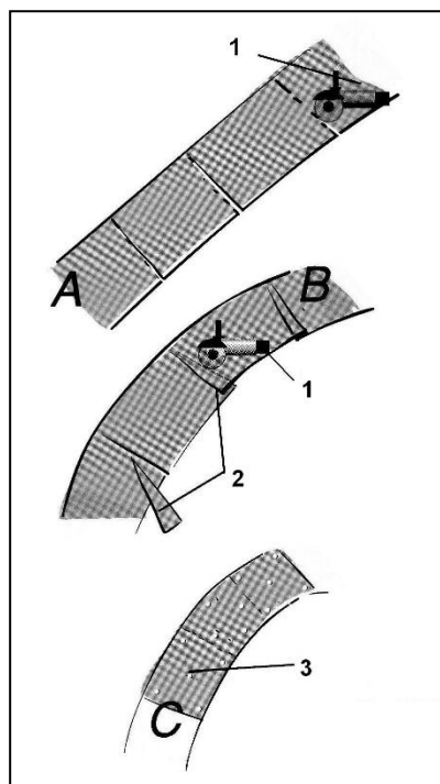
Rys. 1. Siatka z drutu stalowego
