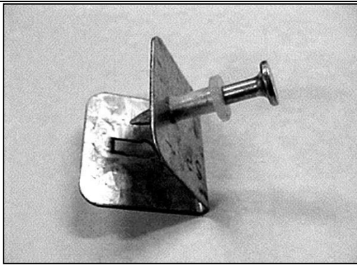
Rys. 5. Klips i kulek do mocowania siatki w podłożu. Klips zakłada się na poprzeczny pręt płaski siatki
