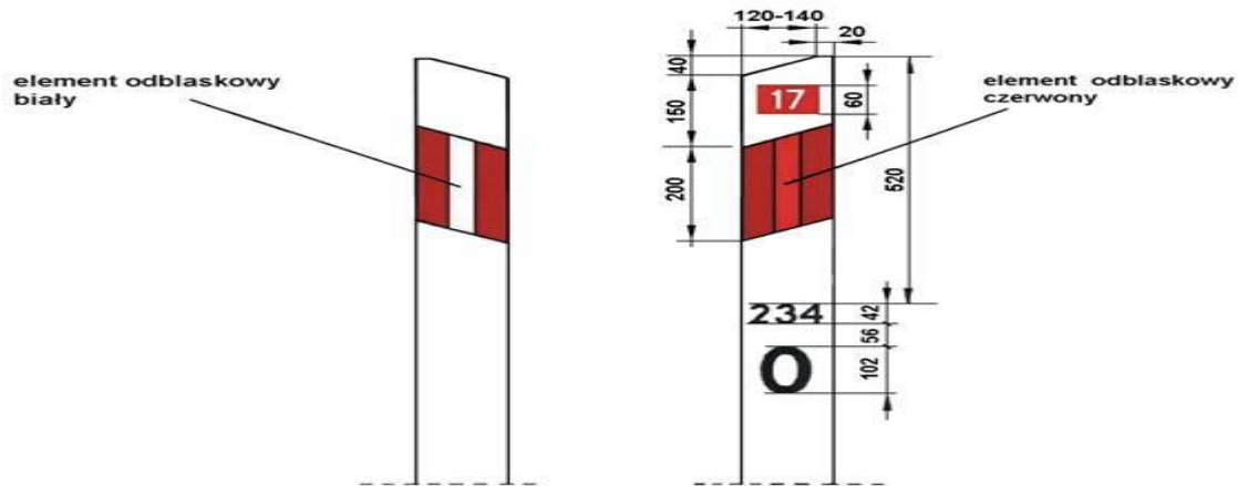
Rys.1. Słupek prowadzący U-1a z naniesionym numerem drogi, znakiem kilometrowym i hektometrowym, przeznaczony do umieszczenia na poboczu drogi, w hektometrze zerowym
