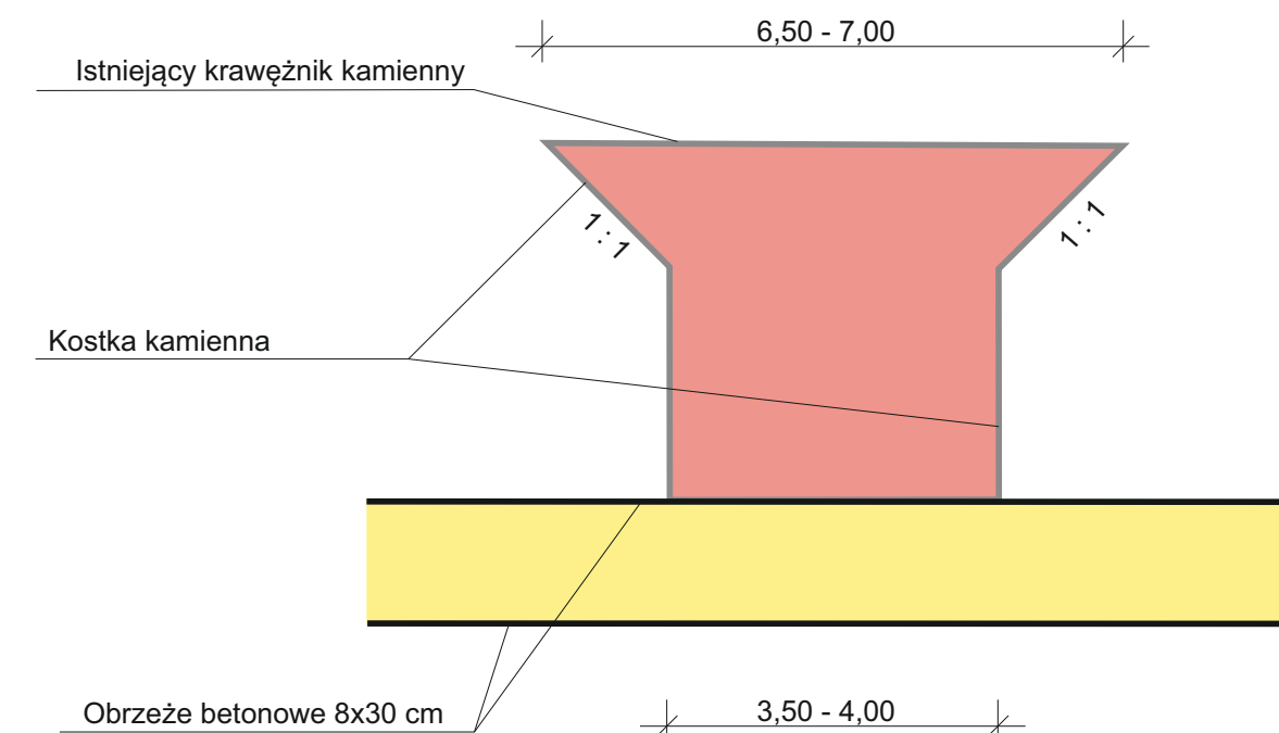
Rzut charakterystyczny zjazdu indywidualnego skala 1 : 100
