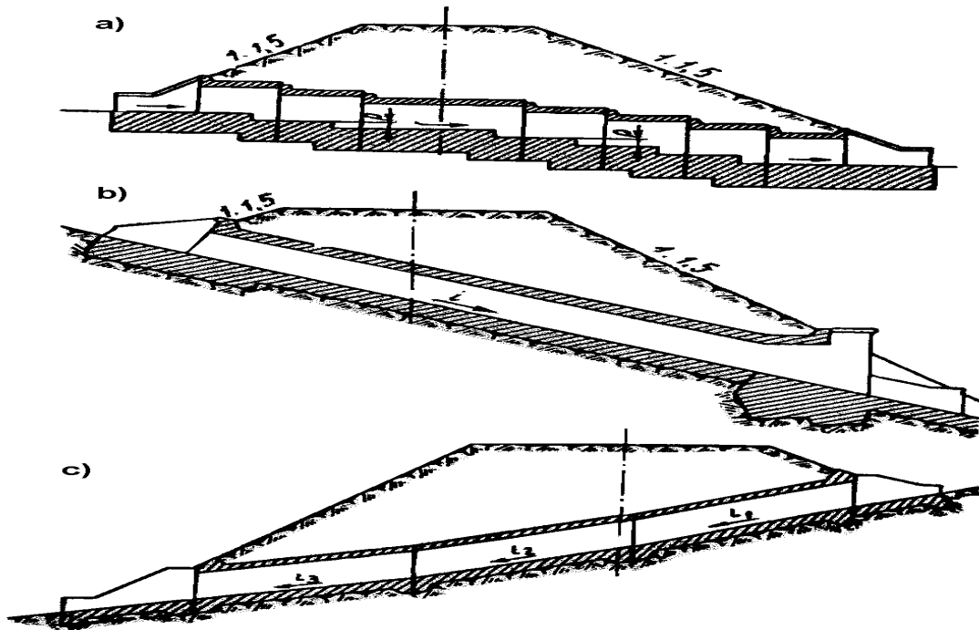
Rys. 3. Progi zabezpieczające przepust przed zamuleniem
