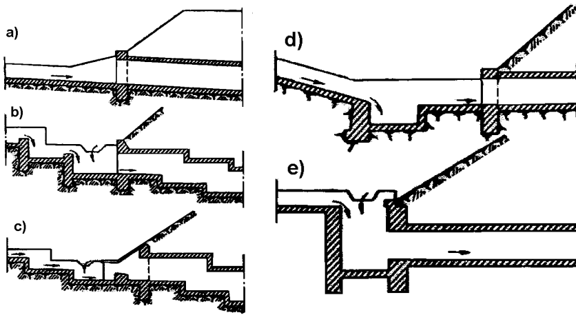
Rys. 2. Przekroje podłużne przepustów na stokach
