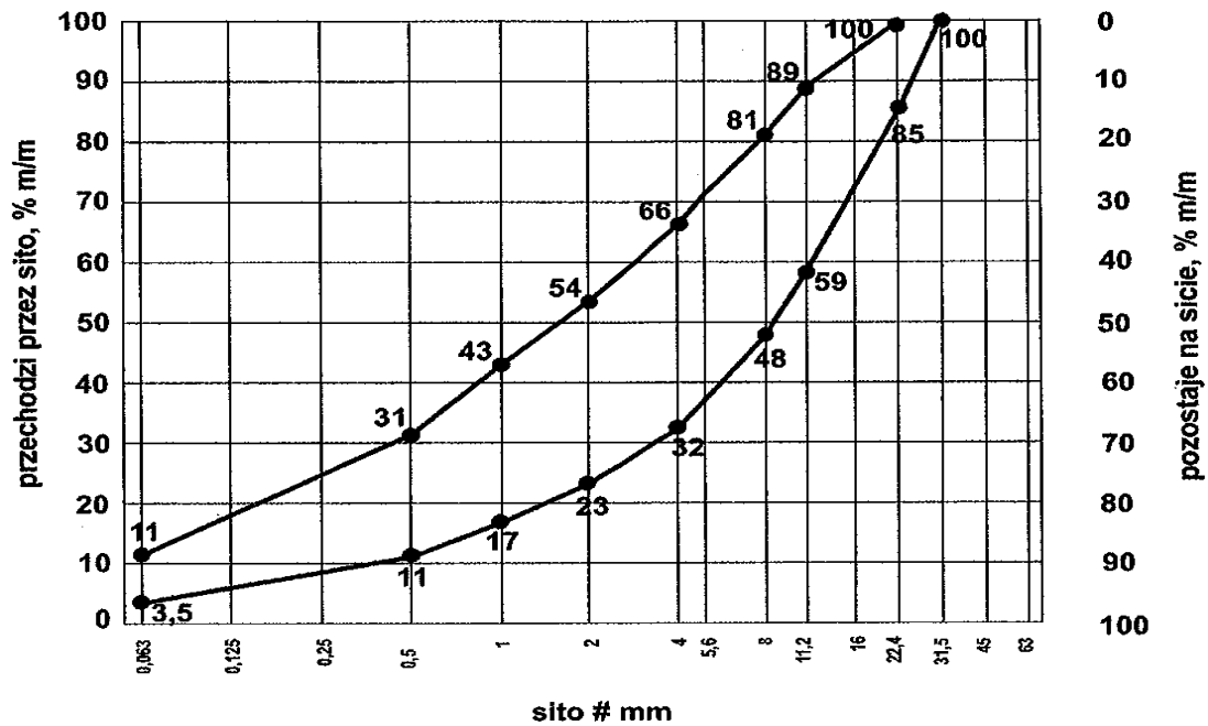
Rys. 2. Krzywe graniczne uziarnienia mieszanki mineralnej 0/22,4 mm
