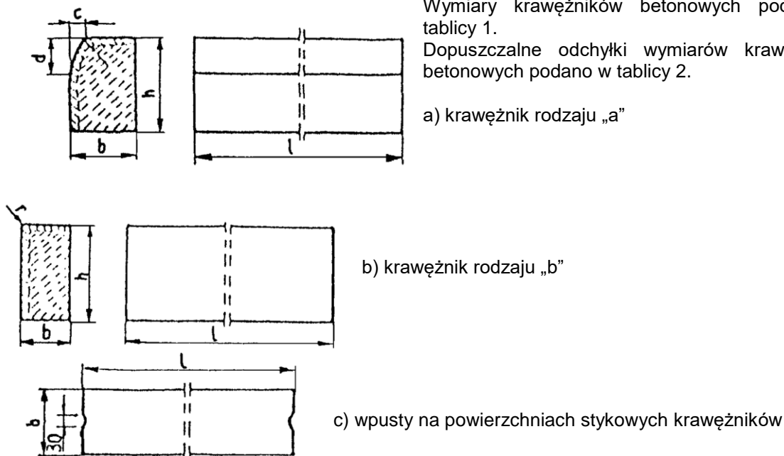
Rys. 1. Wymiarowanie krawężników
