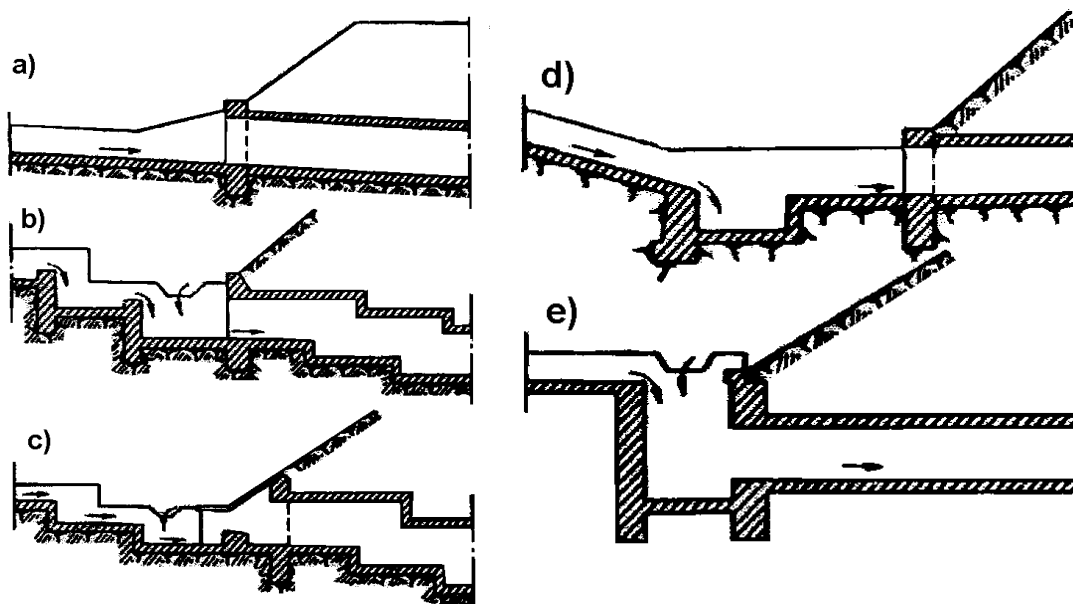
Rys. 2. Przekroje podłużne przepustów na stokach
