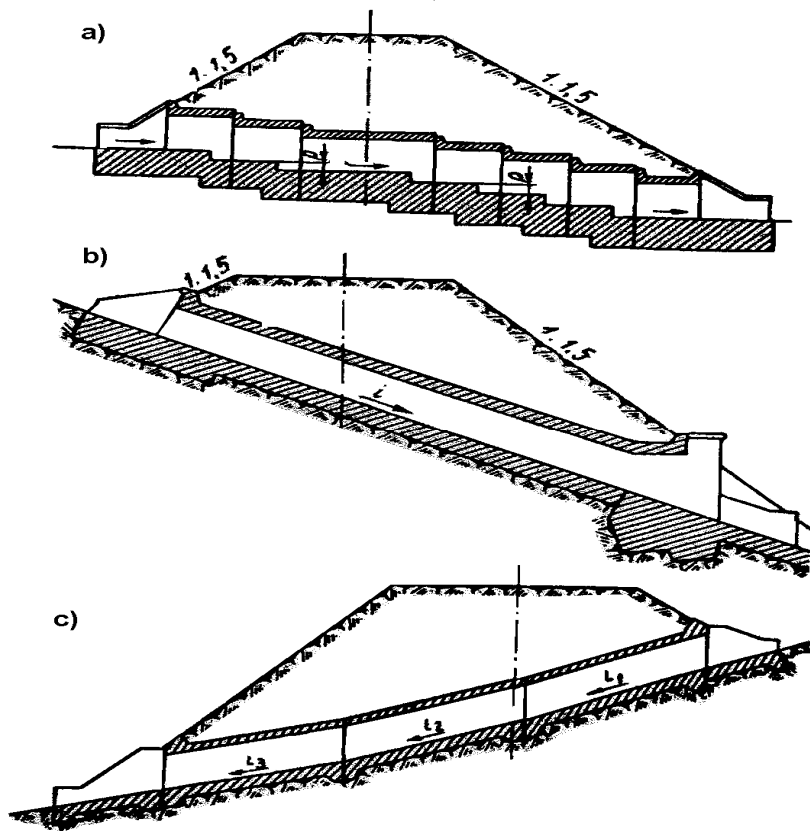
Rys. 3. Progi zabezpieczające przepust przed zamuleniem
