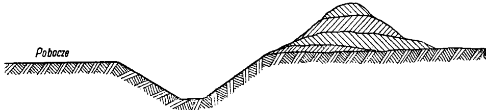
b) Niewłaściwe składanie namułu z oczyszczenia rowu tuż przy skarpie rowu (rów może być zamulony ponownie przez obsuwający się namuł)
