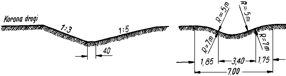
b) Rowy opływowe
