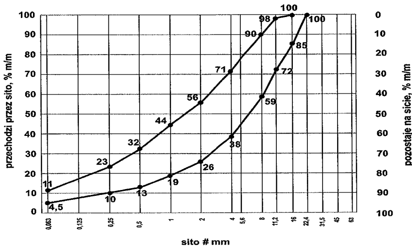
Rys. 3. Krzywe graniczne uziarnienia mieszanki mineralnej 0/16 mm
