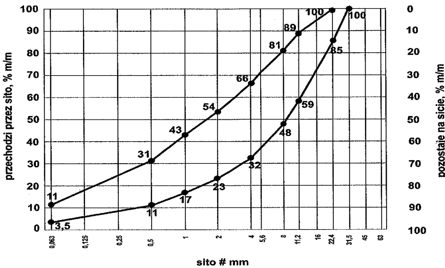
Rys. 2. Krzywe graniczne uziarnienia mieszanki mineralnej 0/22,4 mm
