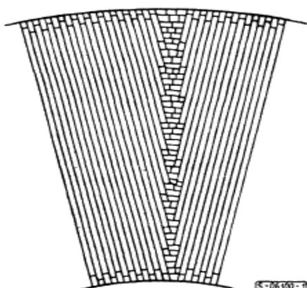
Rys.4. Szczegół układania dużych kostek na łukach
