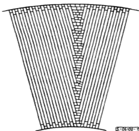
Rys.4. Szczegół układania dużych kostek na łukach
