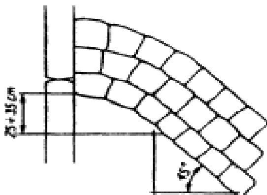
Rys. 3. Zaokrąglenie rzędów kostek przy krawężniku
