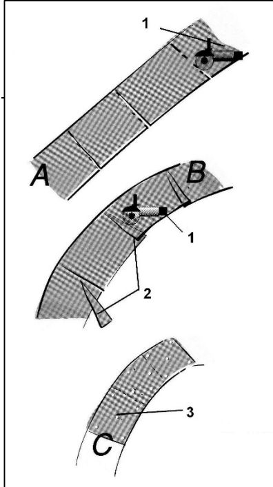
Rys. 2. Ułożenie siatki na podłożu
