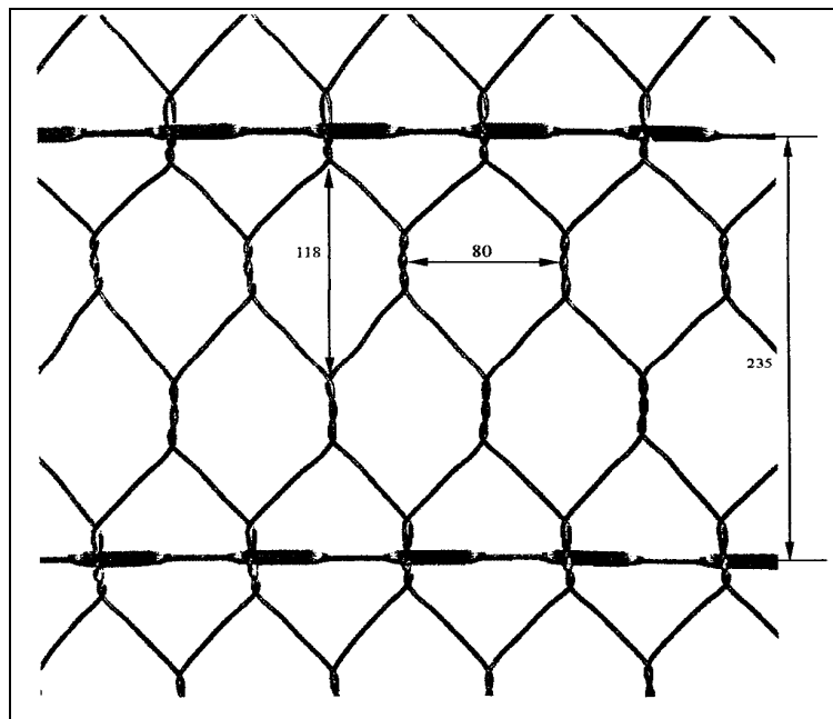
Rys. 1. Siatka z drutu stalowego
