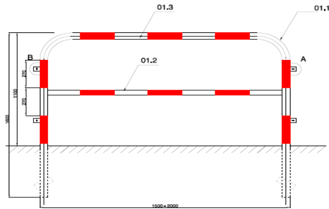
Rys. 1. Wzór bariery ochronnej z rur stalowych U-12a
