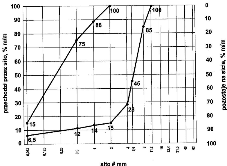
Rys. 2. Krzywe graniczne uziarnienia mieszanki mineralnej 0/11,2 mm
