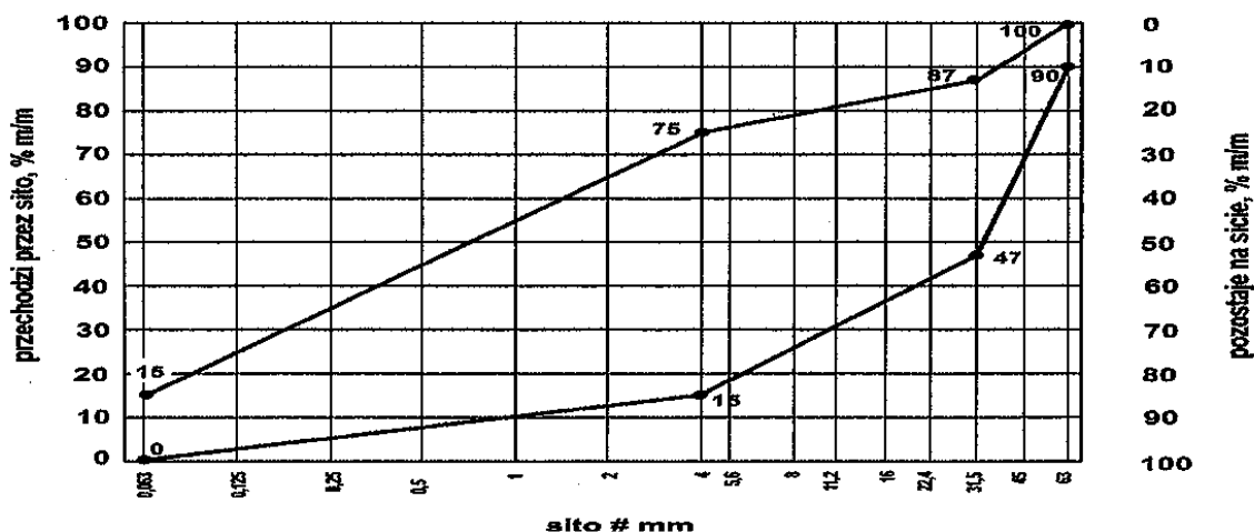
Rysunek 1. Uziarnienie mieszanki 0/63 do warstwy ulepszonego podłoża
