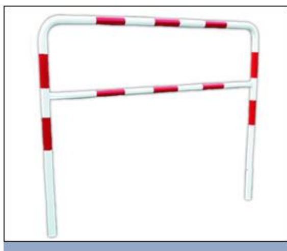
Rys. nr 5 poręcz zabezpieczająca z rur stalowych \varnothing 60 mm, malowanych proszkowo na biało i oklejonych folią czerwoną w pasy biało-czerwone. Szerokość paska czerwonego 15cm, o rozstawie słupków co 2m, H=110 cm
