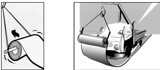
Rys. 2. Ułożenie siatki na podłożu
