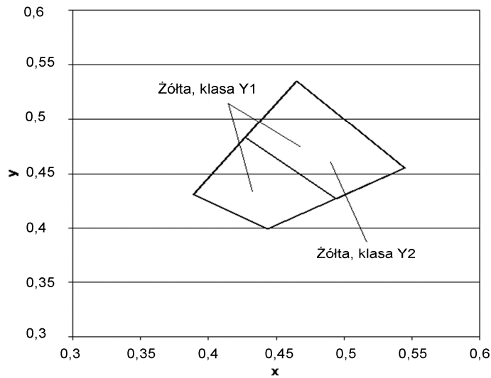
Rys.2. Współrzędne chromatyczności x,y dla barwy żółtej oznakowania
