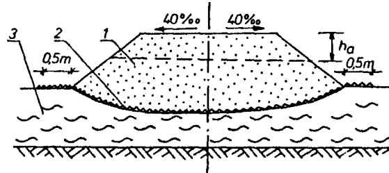
Rys. 2.1. Schemat nasypu na gruncie słabonośnym z zastosowaniem geosynteptyku 1 - nasyp drogowy, 2- warstwa geosynteptyku, 3 - grunt słabonośny
