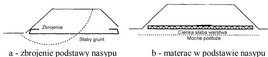
Rys. 2.2. Przykłady zbrojenia nasypów geosynteptykami
