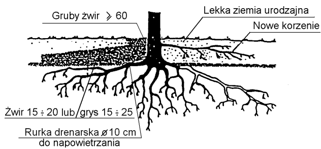
Rys. 3. Pień drzewa obsypany na wysokość 0,2 \div 0,5 m ze specjalnymi napowietrzającymi warstwami żwirowymi (wg [10])
