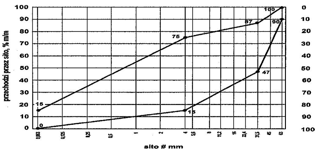
Rysunek 2. Mieszanka kruszyw 0/63 do górnej warstwy podłoża ulepszzonego
